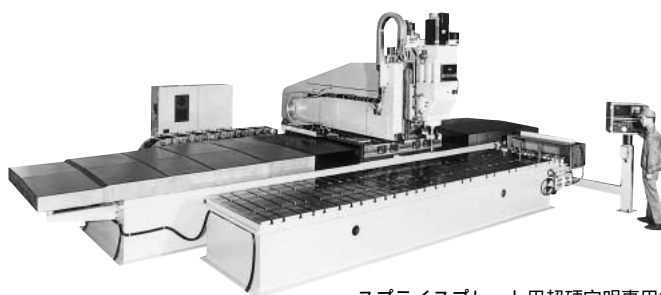
スプライスプレート用超硬穴明専用機 シングルコラム(ATC付) M1S1,000-5,000型
