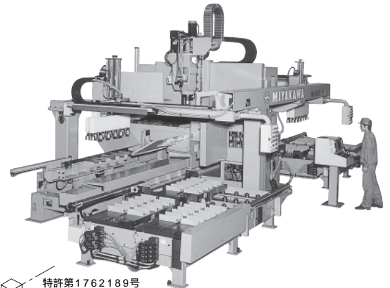
スライスプレート用 つみこみオート穴明機 M1DA500-1200-3P2型
