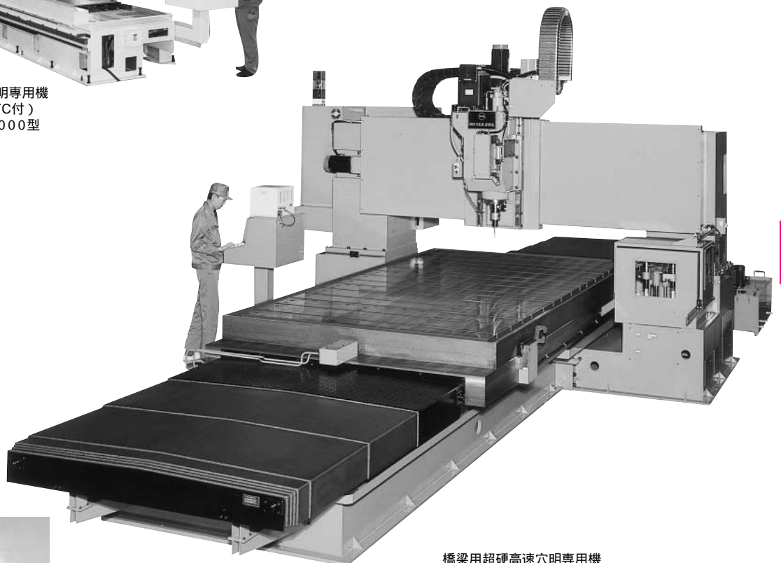
橋梁用超硬高速穴明専用機 ダブルコラム(ATC付) M1D2,000-4,000型
