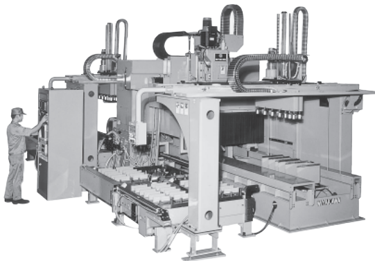
スライスプレート用 つみこみオート穴明機 M1DA500-1200-3P2型
