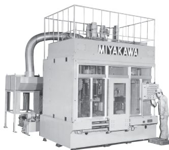
門型多軸ガンドリル・ ガンリーマ専用機
