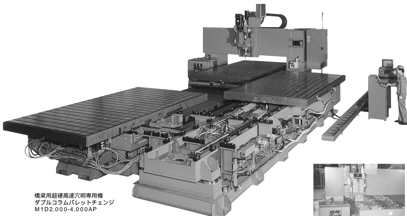
橋梁用超硬高速穴明専用機 ダブルコラムパレットチェンジ M1D2,000-4,000AP
