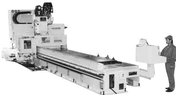
橋梁用超硬高速穴明専用機 ダブルコラム(ATC付) M1DM1,000-5,000型
