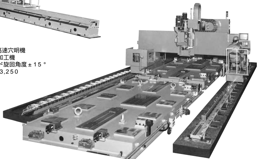
橋梁用超硬高速穴明専用機 NC1軸ガントリー(ATC付) 35-2,000 \times 23,500型
