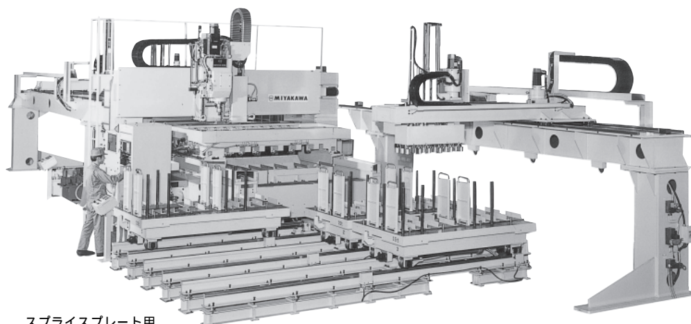
スライズプレート用 つみこみオート穴明機 M1DA650-2000-3P2型
