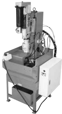
2軸リーマ加工機 ロータリー治具付
