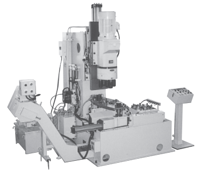
5軸穴明専用機
