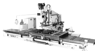
スプライスプレート用超硬穴明専用機 シングルコラム M1S-1,000-3,100型
