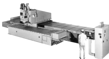
スプライスプレート用超硬高速穴明専用機 シングルコラム(ATC付) M1S1,000-5,000型
