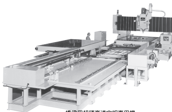
橋梁用超硬高速穴明専用機 ダブルコラムパレットチェンジ M1D2,000-4,000AP
